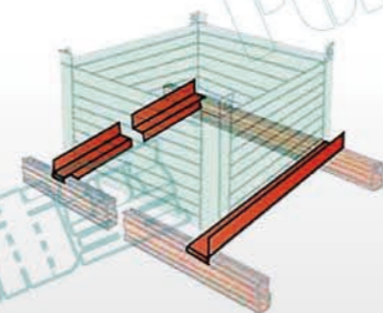
L型跨梁
