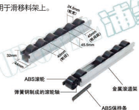
铝合金滚道
